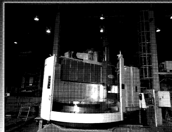
大型NC旋盤 芝浦機械 TUE-200S φ2400
