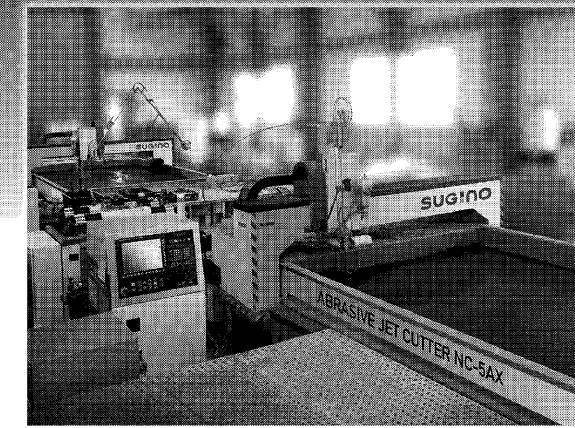
ウォータージェット切断機 280t×2000×4000
