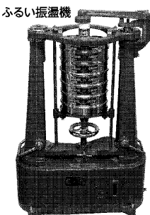
ふるい振盪機
