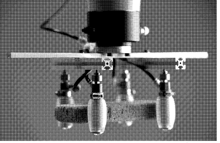
エアを活用したロボットハンド「MKグリッパ」
