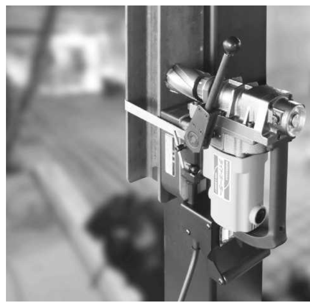
▲磁石で鉄屑などを吸着し、穴位置を固定して穴開けができるドライバー(育良精機提供)
