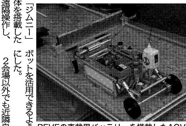
PEVEの車載用バッテリーを搭載したAGV
