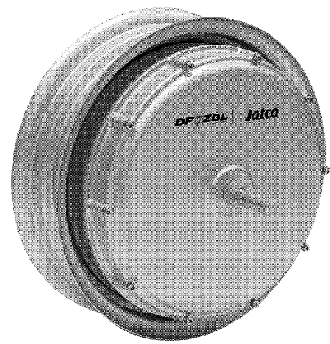
電動バイク向け2速自動変速インホイールモータードライブユニット
