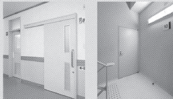
自動閉鎖装置付引戸「カムスライダー」 環境配慮型スチールドア「SGD」
