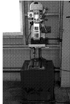
主軸の即時停止機能を備えた遠州工業のボール盤
