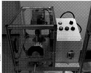
軍手の巻き込まれ事故を再現する装置「BT-100」
