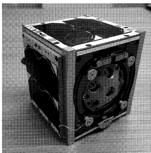
小型人工衛星（中央）を搭載した小型人工衛星
